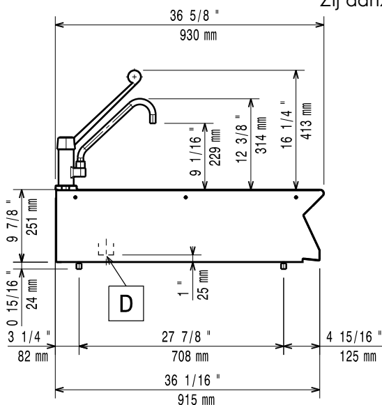
Zij aanzicht
